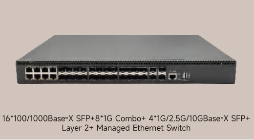
LT-S8328XG-4XS16GX8GC
